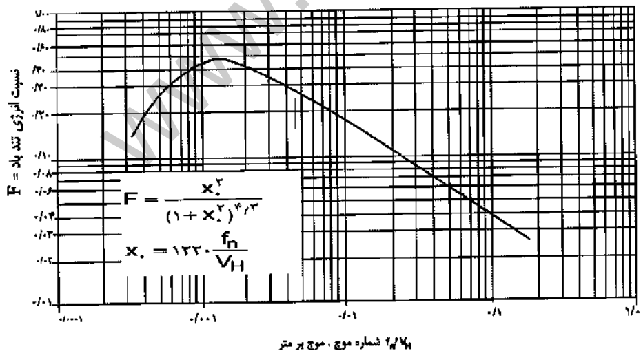
شکل پ-۴-۶-۳ نسبت انرژی تند باد (F)
