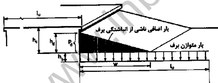
شکل ۷-۸-۶ نمایش برف انباشته شده بر بام پایین‌تر
