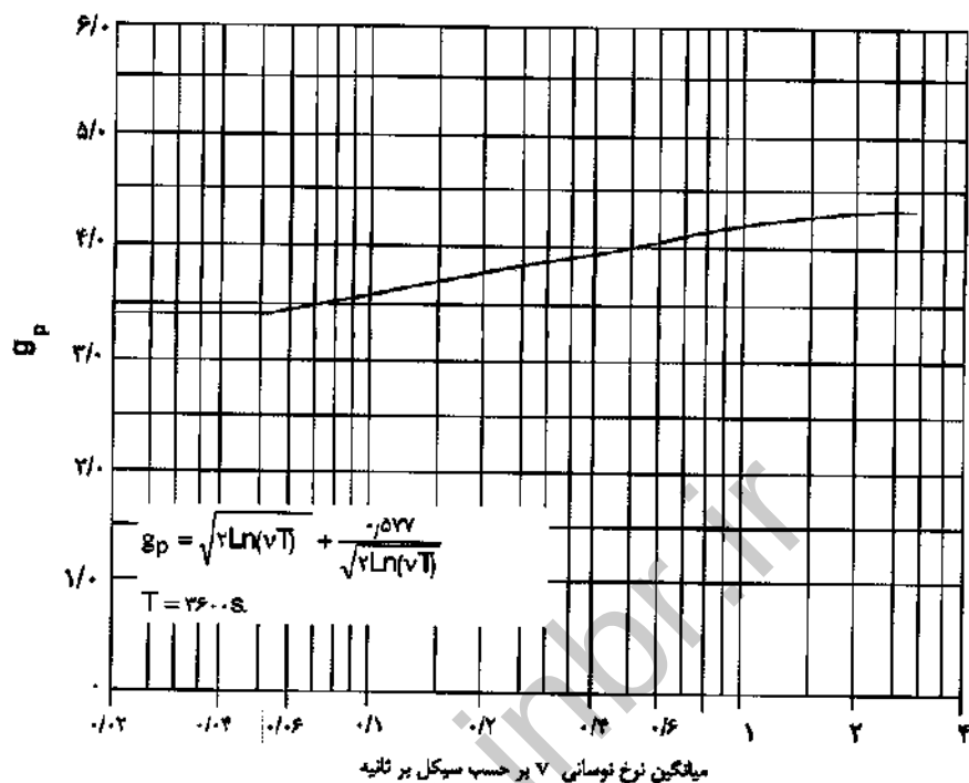
شکل پ-۴-۴-۴ ضریب پیشینه آماری بار ( G_p )
