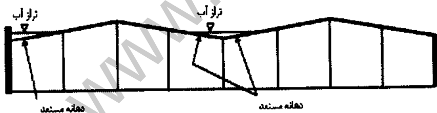
شکل ۸-۶-۲ دهانه‌های مستعد برای انباشتگی آب و کنترل ناپایداری با شیب بام ۲٪ یا بیشتر
