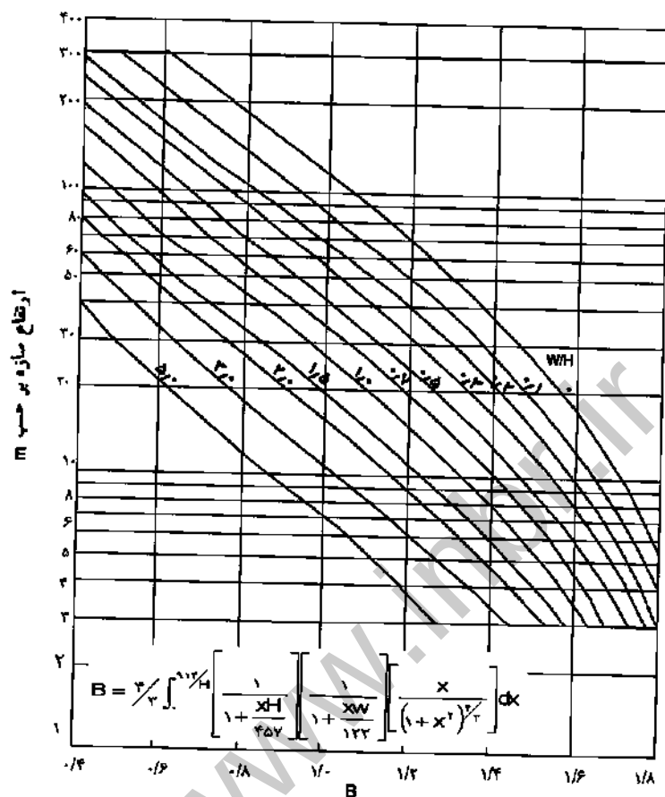
شکل پ-۶-۴-۱ ضریب آشفته‌گی محیط ساختمان (B)
