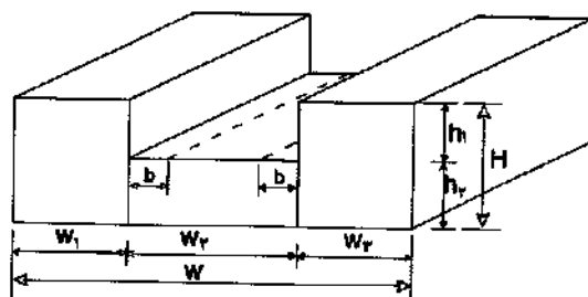
شکل ۱۰-۱۰-۶ نسبت ابعادی ساختمان‌های با بام پله‌ای تخت
