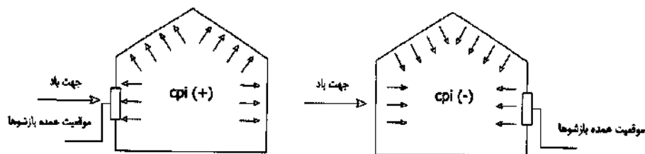
شکل ۶-۱۰-۱۲ ضریب اثر بارشو C_{pi}
