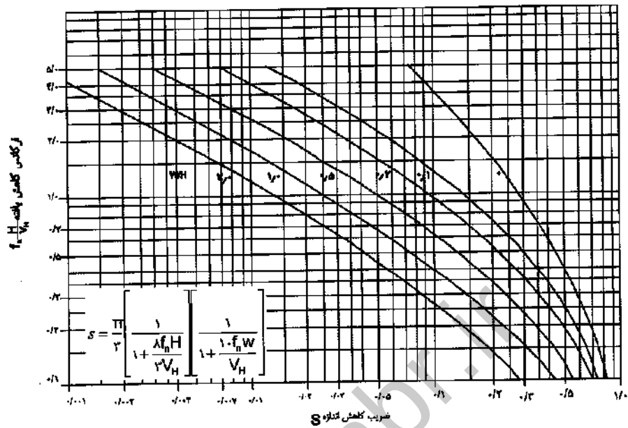
شکل پ-۴-۶-۲ ضریب کاهش اندازه (S)
