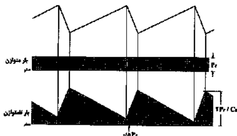
شکل ۴-۷-۶ بار متوازن و نامتوازن در بام های دندانه دار
