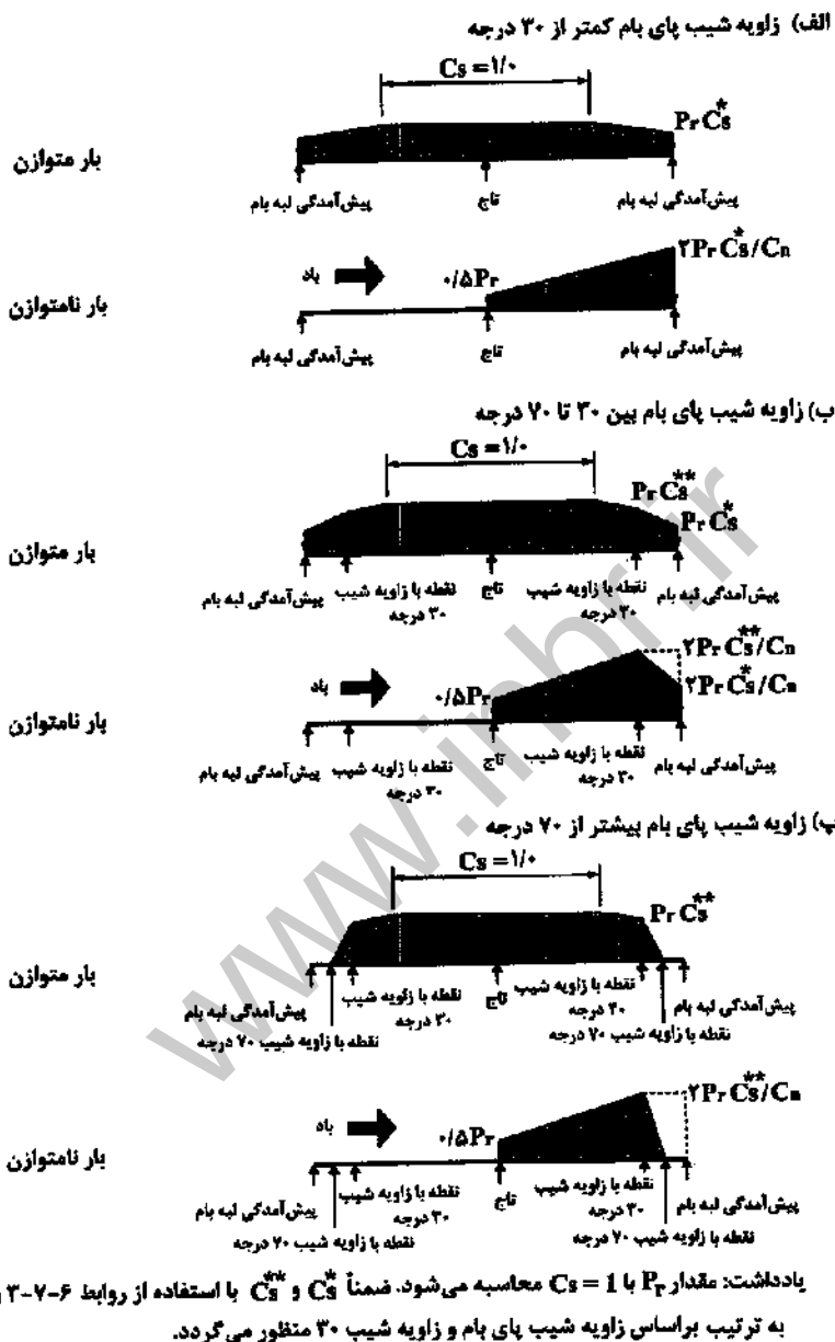
شکل ۶-۷-۳ بار متوازن و نامتوازن در بام های قوسی
