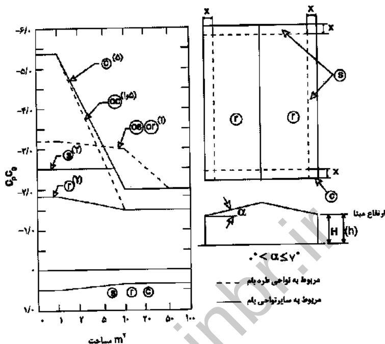
شکل ۶-۱۰-۶ ضرایب ترکیبی فشار و مکش خارجی C_p C_g برای طراحی پوشش‌ها و اجزاء بام (با زاویه شیب کمتر از ۷ درجه، یا بدون طره)
