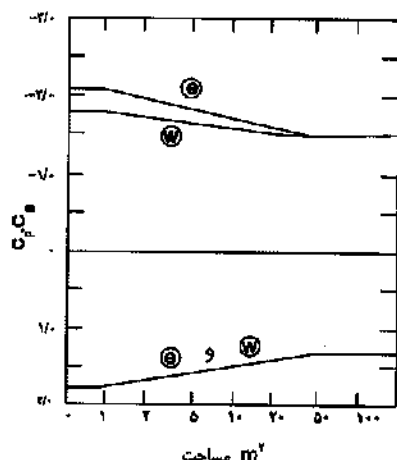
شکل ۵-۱۰-۶ ضرایب ترکیبی فشار و مکش خارجی C_p C_g برای طراحی دیوار و پوشش نما
